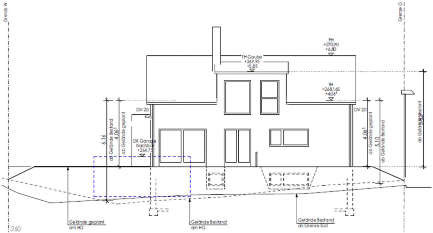
Ansicht Süd
