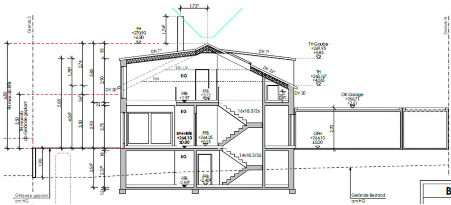
Schnitt
